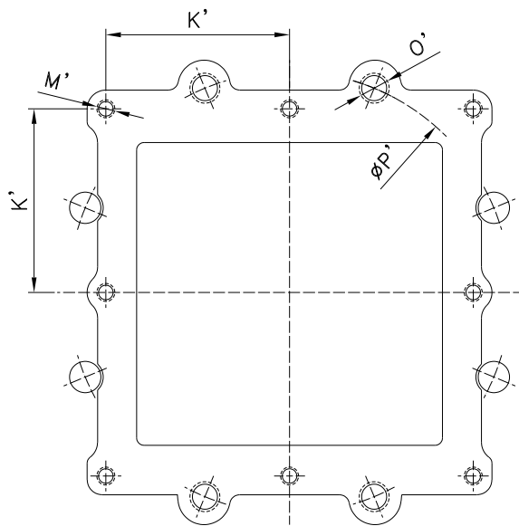
DN 100 - 250 DN 4" - 10"
